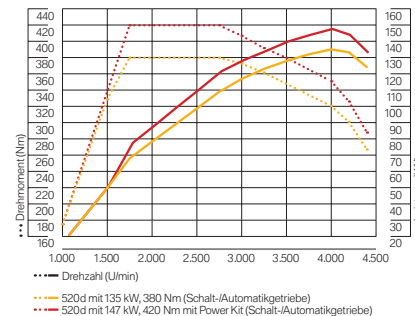
5 Leistungswerte des BMW 520d mit BMW M Performance Power Kit Vollast 520d
