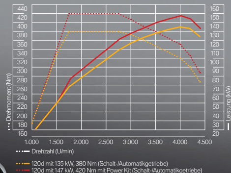
Leistungswerte des BMW 120d mit BMW M Performance Power Kit Vollast 120d
